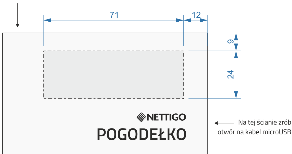
Spód pudełka. Położenie otworu pod wyświetlacz
